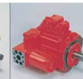
斜板形アキシャル ピストンポンプ Swash plate type axial piston pump K3VG series (P2-3参照)
