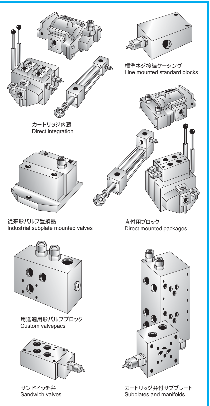
バルブブロック/Valve blocks
